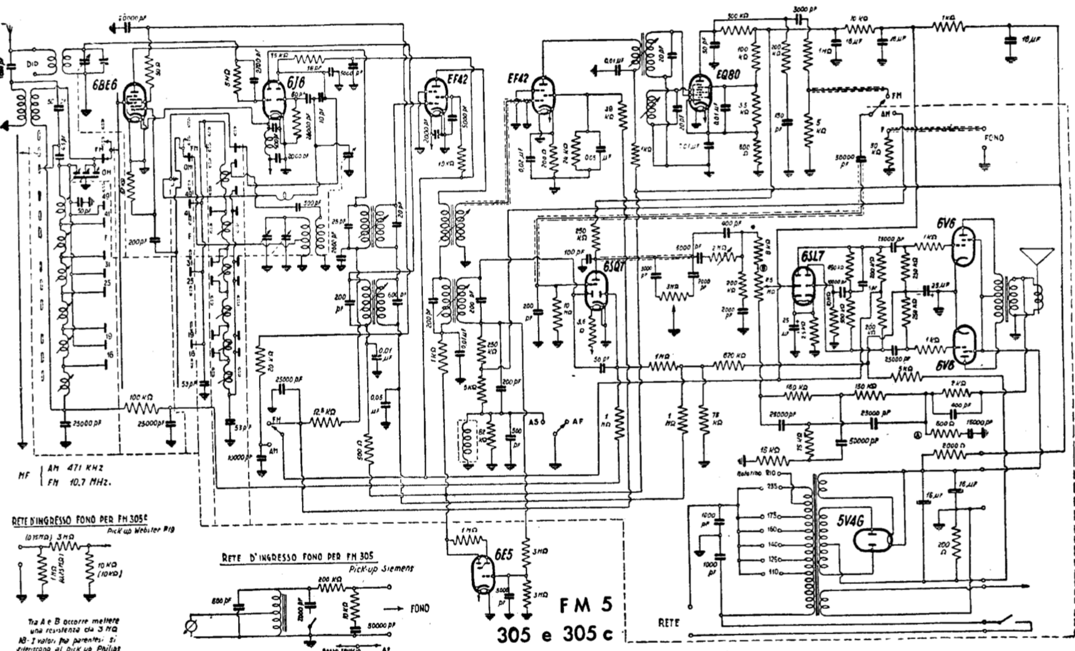
MAGNADYNE RADIO - Mod. FM5 e modelli derivati 305 e 305 c - A modulazione d'ampiezza e di frequenza, con enneodo EQ80 per la rivelazione FM. La rivelazione AM è ottenuta con una 6SQ7, la quale provvede anche alla preamplificazione BF. BF. Medie frequenze 471 kc e 10,5 Mc. Potenza d'uscita 10 watt indistorti.
